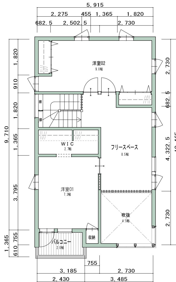
2階平面図
