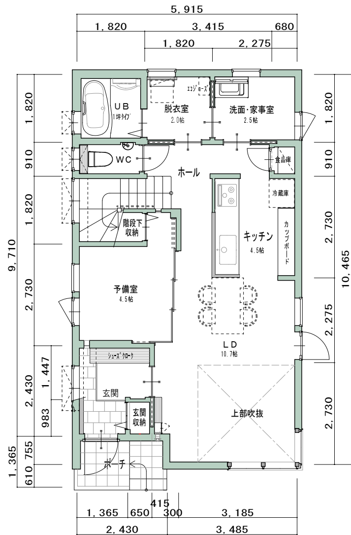
1階平面図
